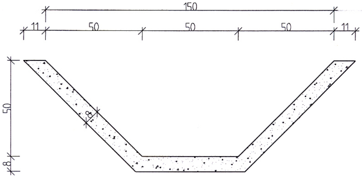
Sezione tipo sc. 1/10
