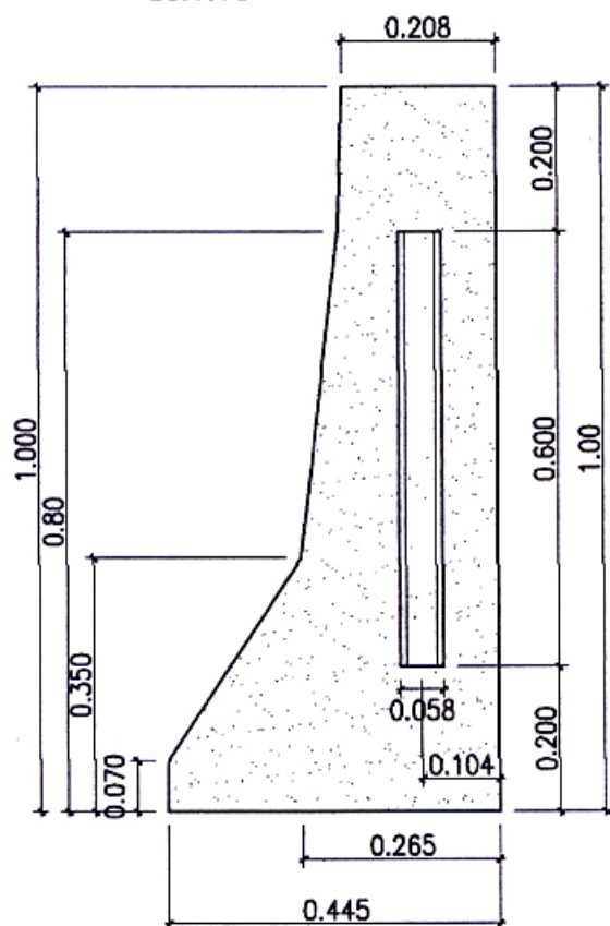
Prospetto Laterale
