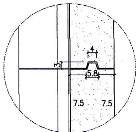
Particolare Innesto ad incastro
