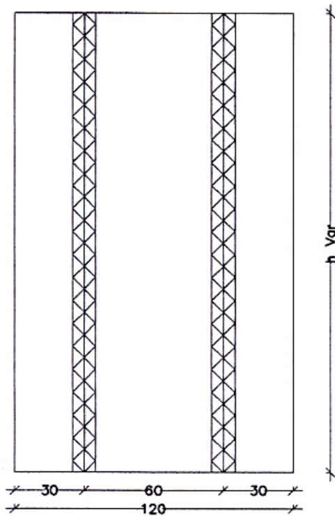
Pianta sc. 1/20
