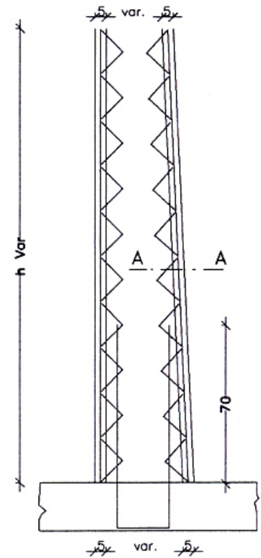
Sezione sc. 1/20
