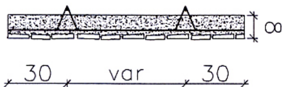
Sezione tipo
