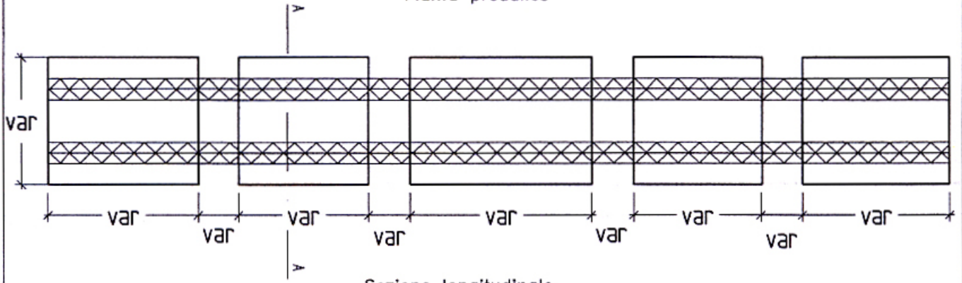
Sezione longitudinale
