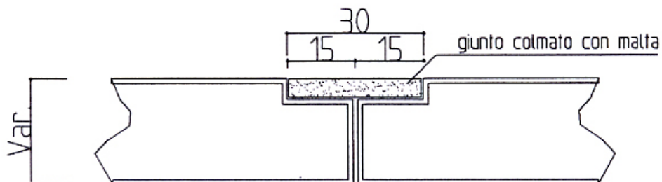
PARTICOLARE GIUNTO A PAVIMENTO
