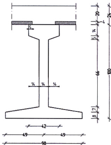
Sezione tipo trave
