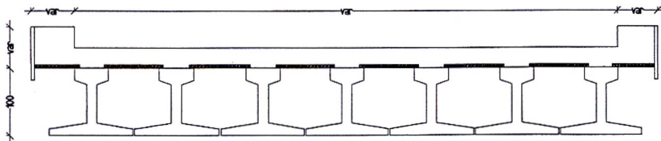
Sezione Tipo Impalcato
