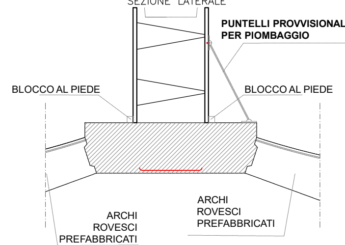
SEZIONE LATERALE
