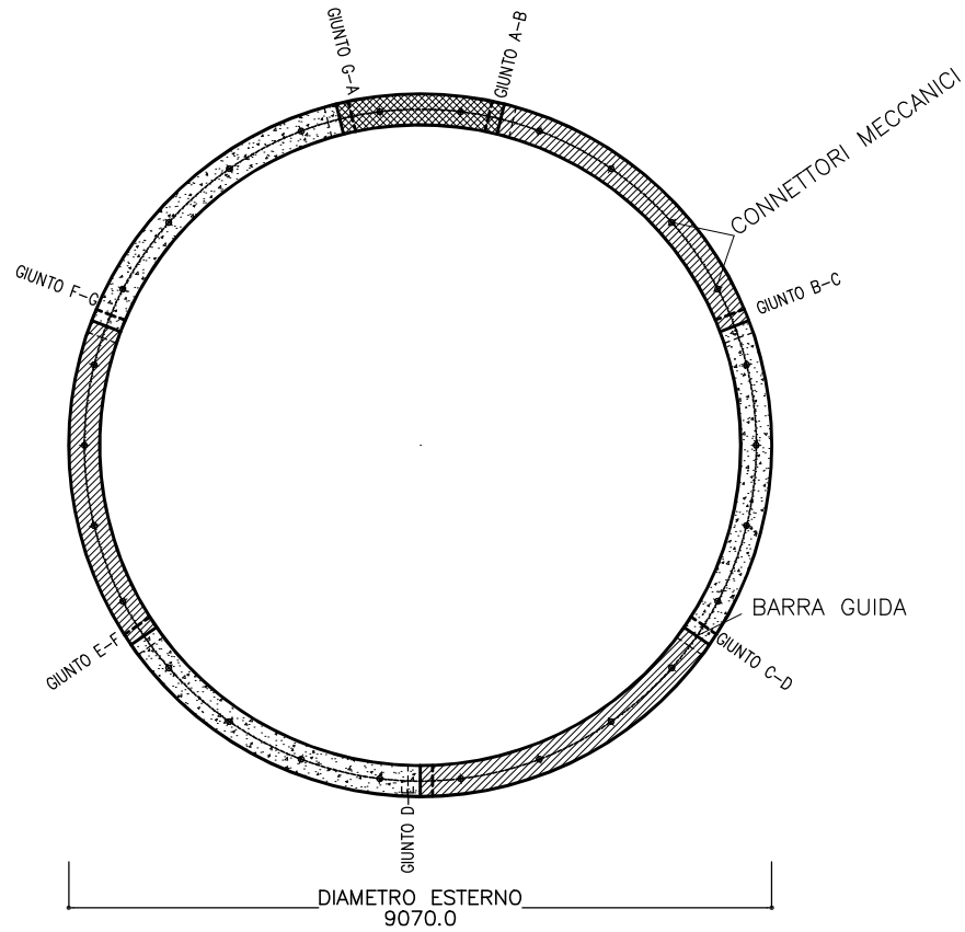
SEZIONE TRASVERSALE CONCIO
