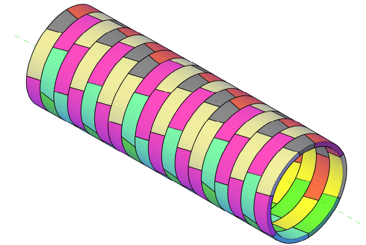
VISTA ASSONOMETRICA FUORI SCALA
