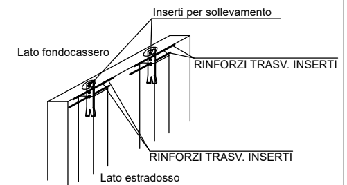
VISTA PROSPETTICA
