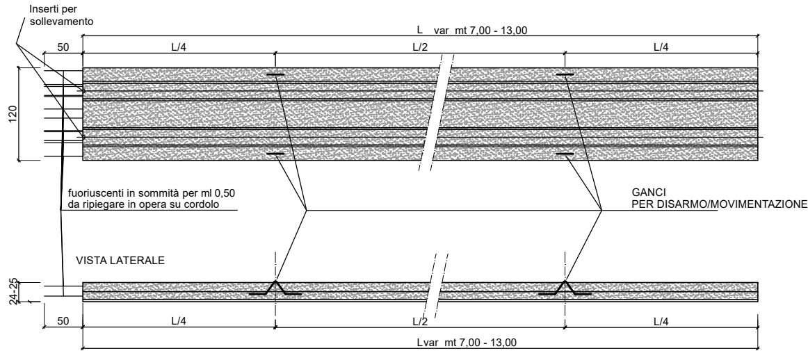
PROSPETTO POSTERIORE
