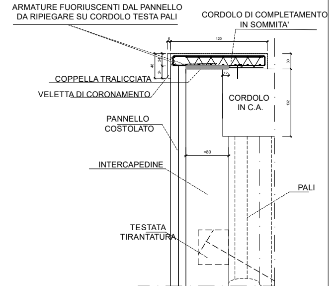
SEZIONE TRASV. IN OPERA
