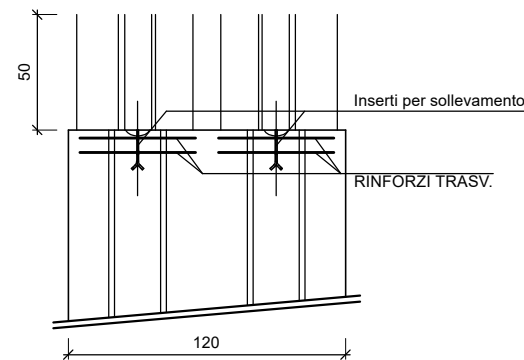
DETTAGLIO SOMMITA' PANNELLO PROSPETTO
