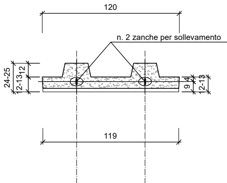
SEZIONE TRASV. - CARPENTERIA
