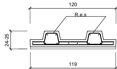
SEZIONE TRASV. - ARMATURA
