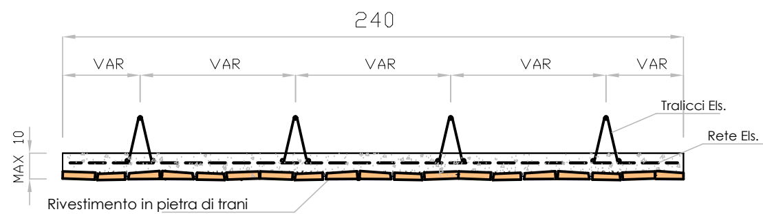
Sezione Trasv.
