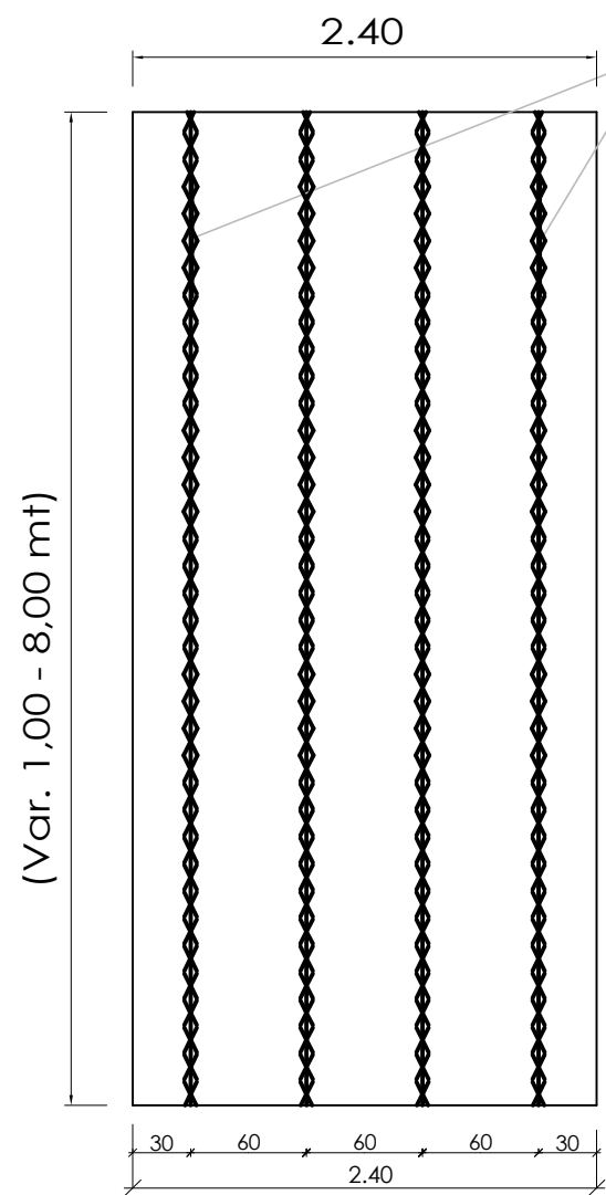
Prospetto Posteriore
