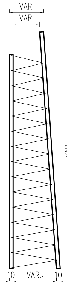
PROSPETTO PARETE INTERNA
