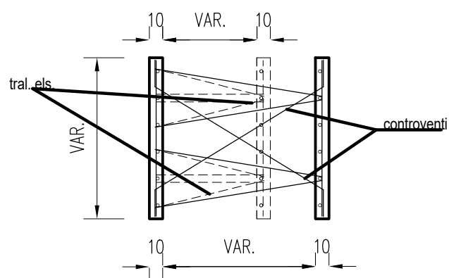
SEZIONE VERTICALE
