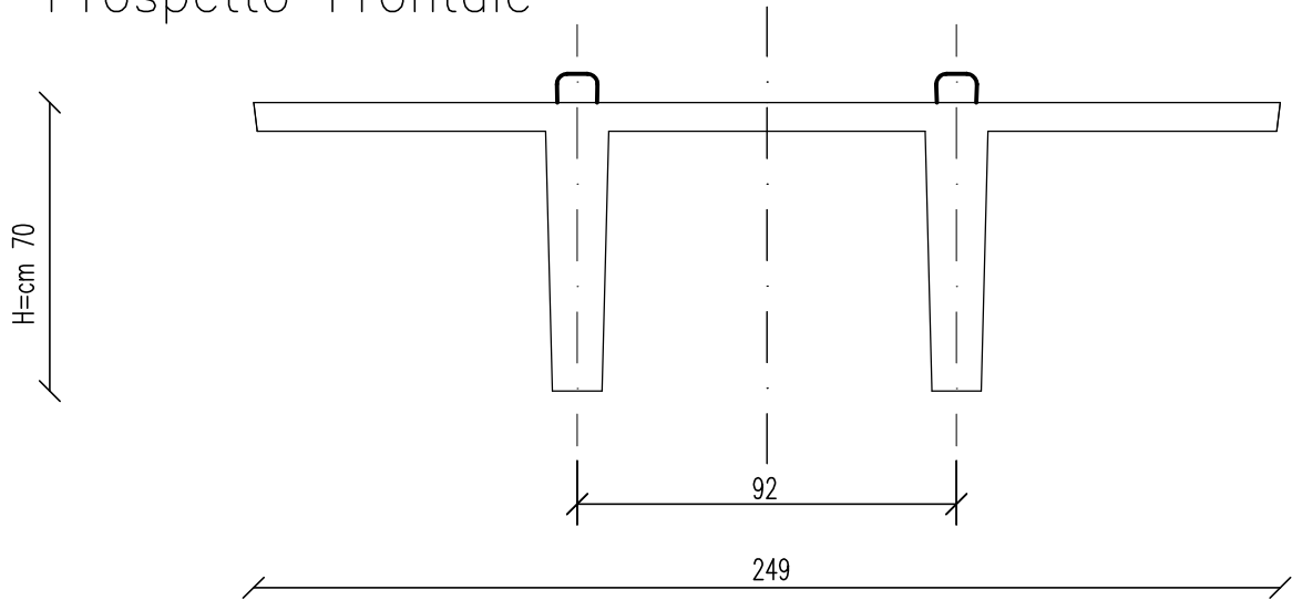
Prospetto Frontale
